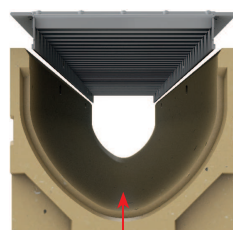
V-Průřez
